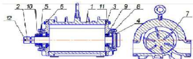
1. Корпус; 2. Ротор; 3. Кришка; 4. Кришка; 5. Кришка; 6. Кришка; 7. Лопатка; 8. Підшипник; 9. Манжета; 10. Манжета; 11. Ущільнює гумове кільце; 12. Шпонка.
